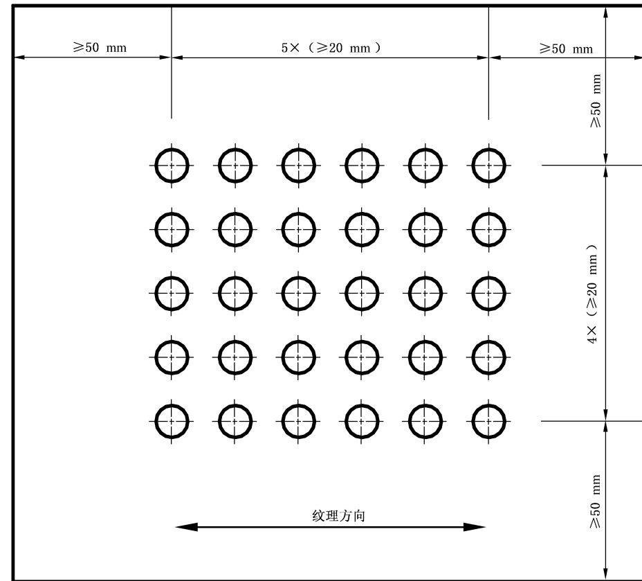
图2 试件冲击部位的确定
